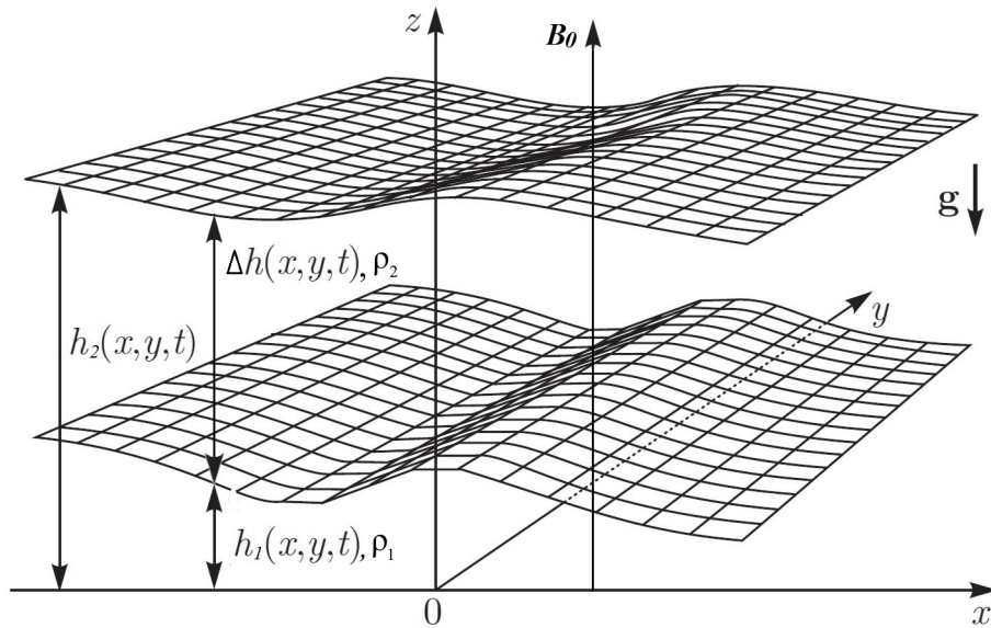
Рис. 1: Тонкий слой плазмы в вертикальном магнитном поле, разделенный на два слоя различной, но постоянной плотности.
